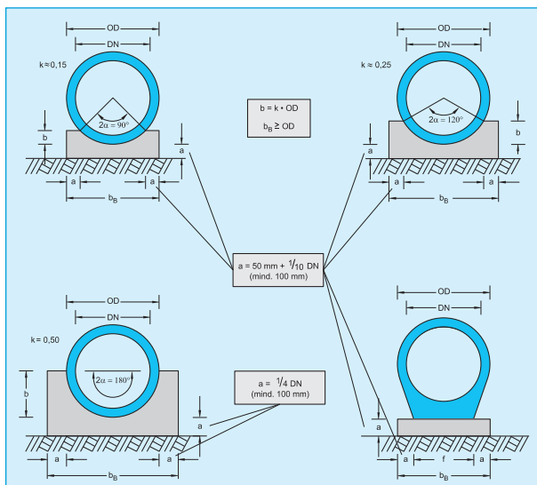
Bild 4: Bettung auf Beton (Beispiele für übliche Auflagerwinkel)
