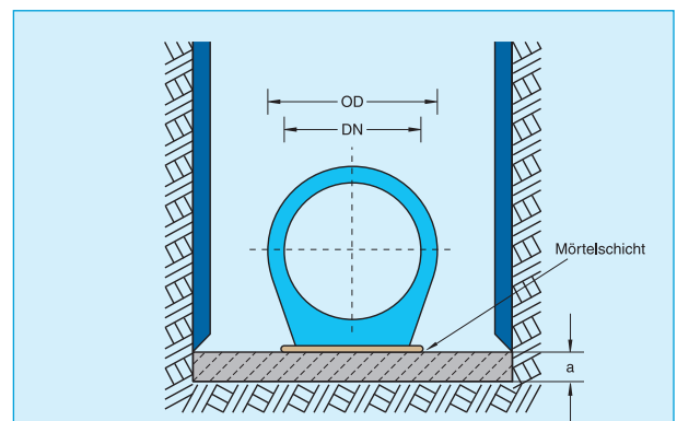
Bild 7: Betonbettung für Rohre mit Fuß auf Mörtelschicht a = 50 \text{ mm} + 1/10 \text{ DN} , min a = 100 \text{ mm}
