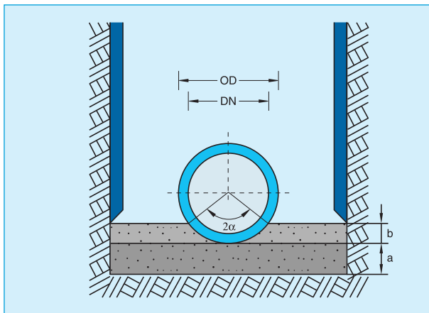
Bild 3: Bettung Typ 1 (Regelausführung) bei normalen Böden: a = 100 \text{ mm} + 1/10 \text{ DN} in mm bei festgelagerten Böden oder Fels: a = 100 \text{ mm} + 1/5 \text{ DN} , min a = 150 \text{ mm}
