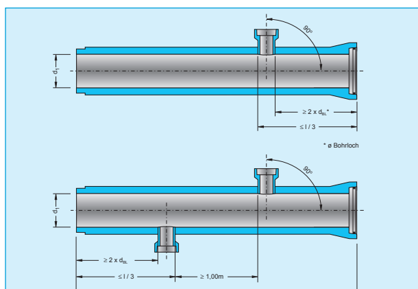
Bild 12: FBS-Rohre mit unterschiedlicher Anordnung von Abzweigen
