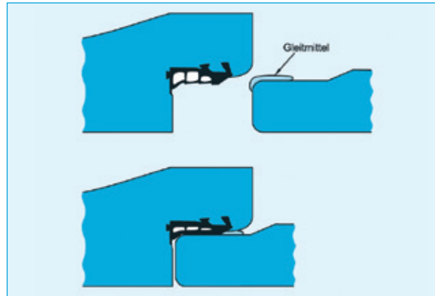
Bild 9a: Werkseitig fest in die Muffe eingebaute Gleitringdichtung
