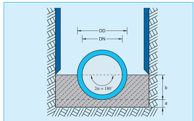
Bild 6: Betonbettung 180^\circ a = 1/4 \text{ DN} , min a = 100 \text{ mm}
