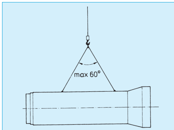
Bild 1: Spreizwinkel bei Seil- und Kettengehängen
