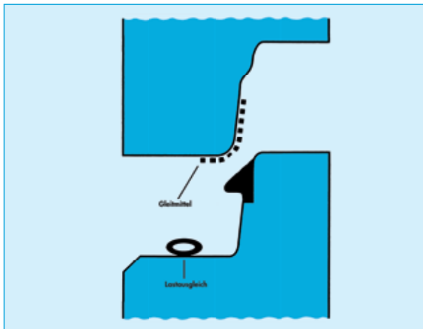
Bild 10b: Schacht
