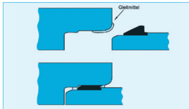
Bild 10a: Werkseitig auf dem Spitzende fixierte Gleitringdichtung
