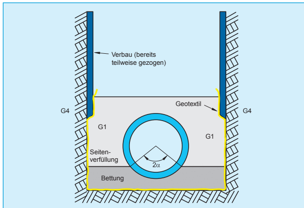
Bild 8: Schutz gegen Ausspülen des Auflagers und des anstehenden Bodens durch Geotextil
