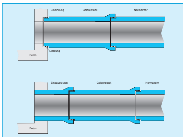
Bild 11: Mögliche Varianten eines Rohranschlusses an ein Bauwerk
