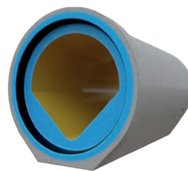
Duoliner Rohrsystem mit Drachenprofil
